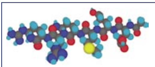
Třírozměrný vzorec heptapeptidu
